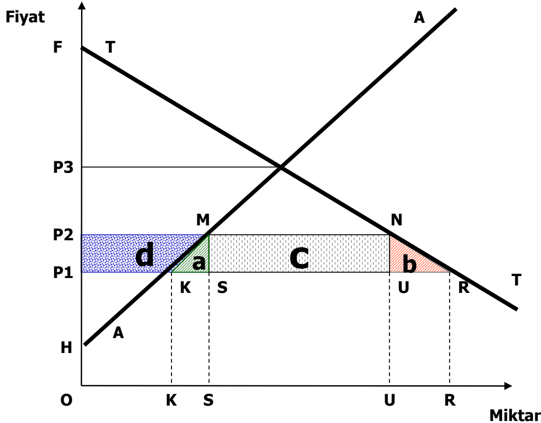
Grafik 1: Gümrük Vergilerinin Kısmi Denge Etkileri
