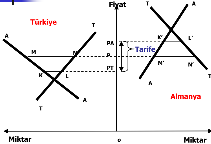
Grafik 4: Gümrük Vergisinin Yansımaları
