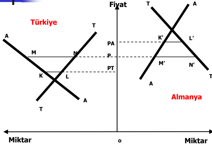
Grafik 4: Gümrük Vergisinin Yansımaları
