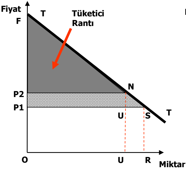
Grafik 2: Tarifelerin Rant Etkileri
