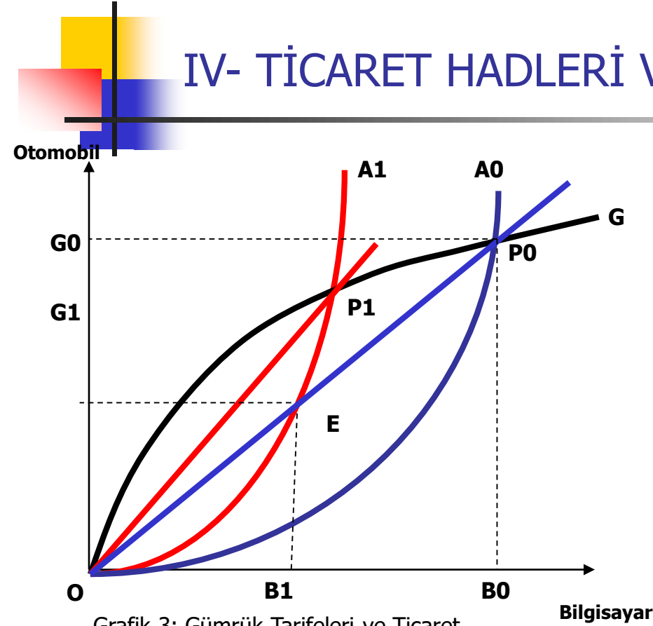
Grafik 3: Gümrük Tarifeleri ve Ticaret Hadleri
